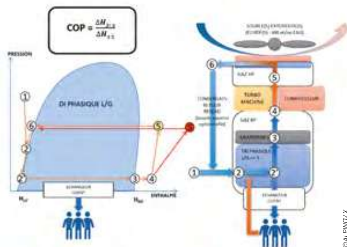
Procédé de génération de froid ALPINOV X
