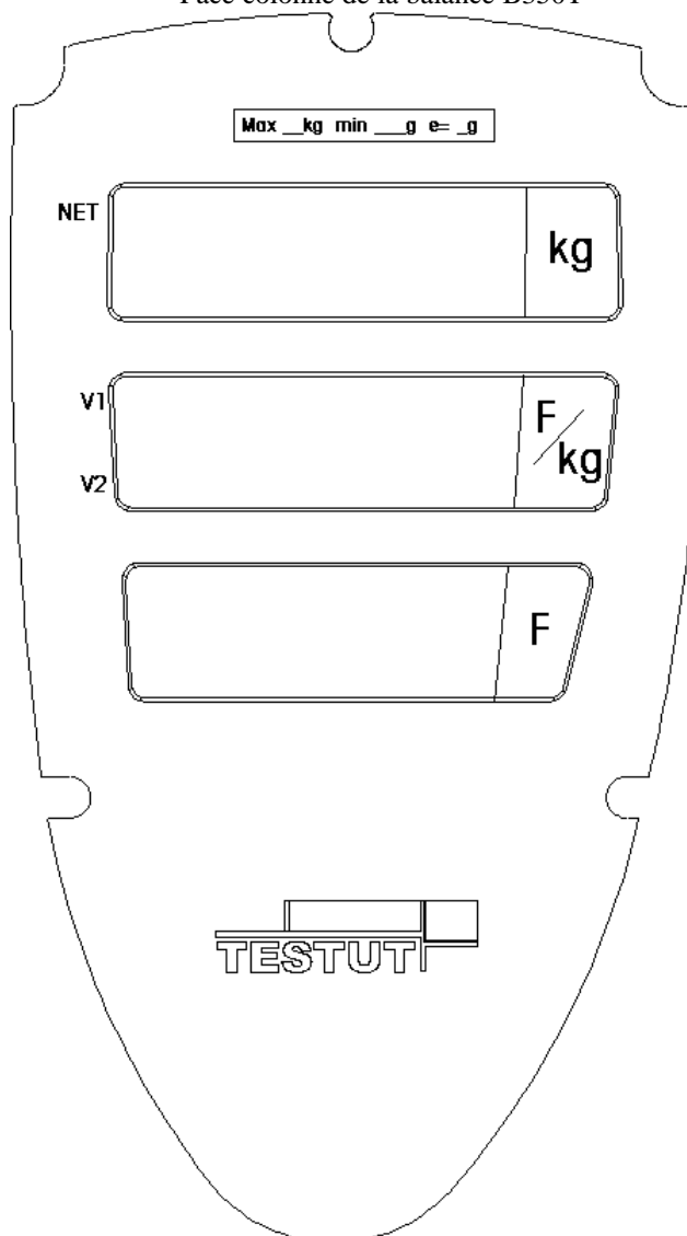
Face colonne de la balance B350T
