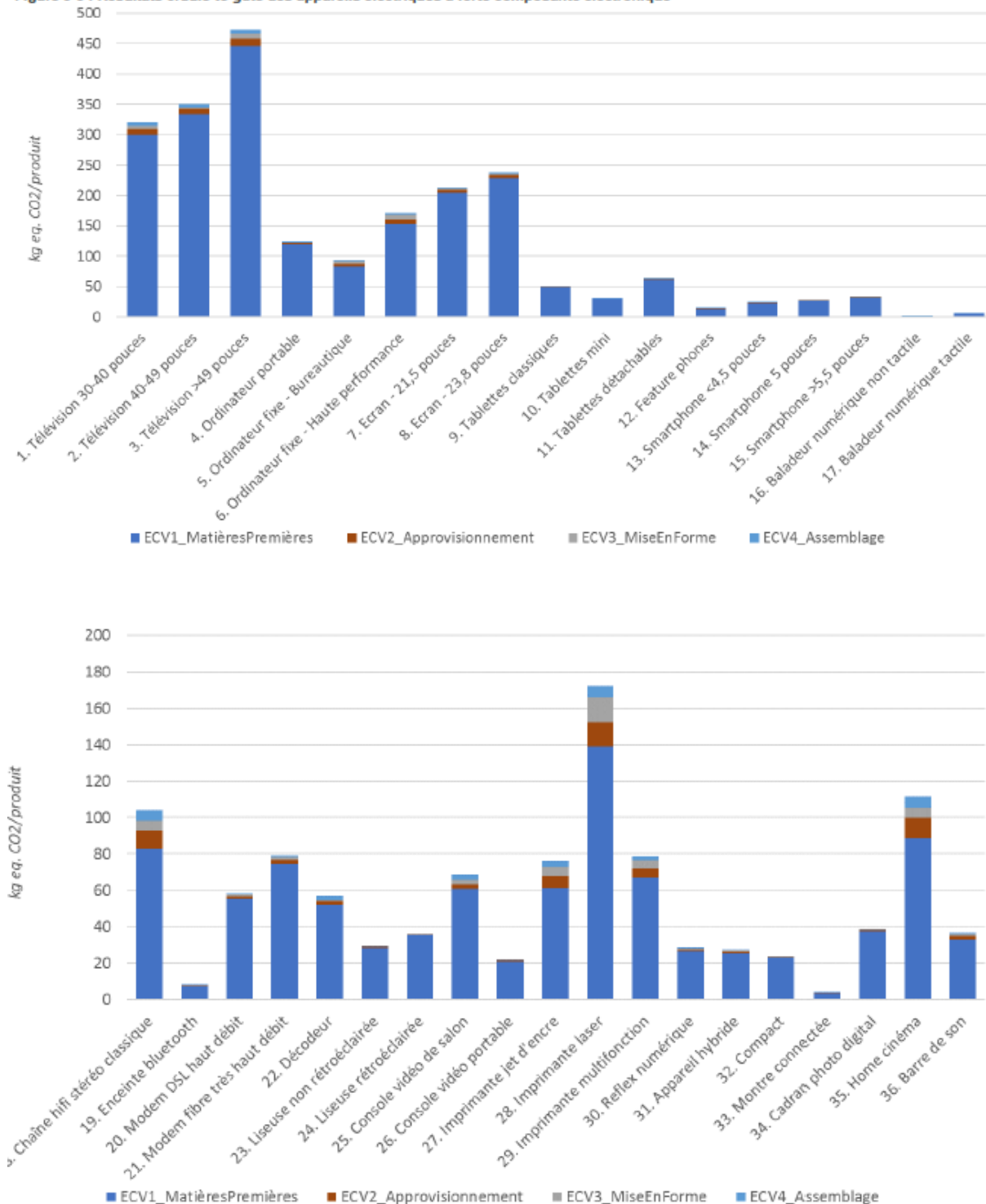
Figure 5-3 : Résultats cradle-to-gate des appareils électriques à forte composante électronique
